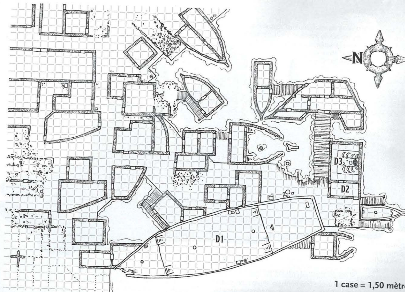
CARTE 4.2 : RIVEBRUME
