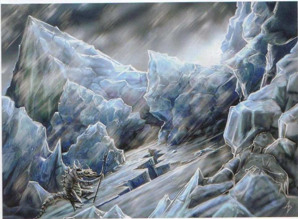
Cania
