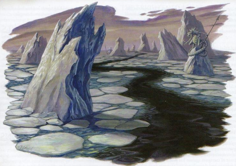
Stygia
