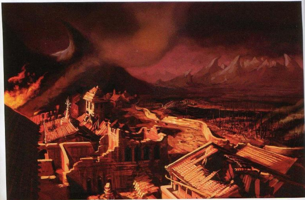
Maladomini
