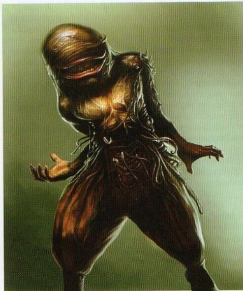
A kalabon
