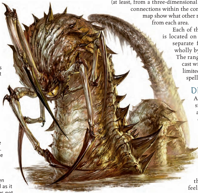
Golothoma
